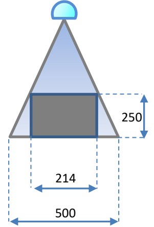
Işın Diyagramı (mm)
